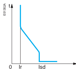
Zabezpieczenie przeciążeniowe oraz zwarcia bezwzględne
