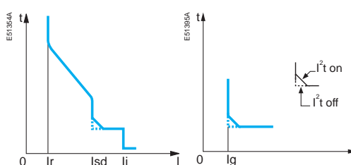
Zabezpieczenie przeciążeniowe oraz zwarcia zwłoczne i bezwzględne
