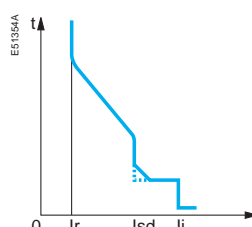
Zabezpieczenie przeciążeniowe oraz zwarcia zwłoczne i bezwzględne
